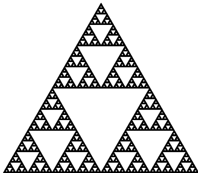
Figur 3: Sierpinski-trekanten.
